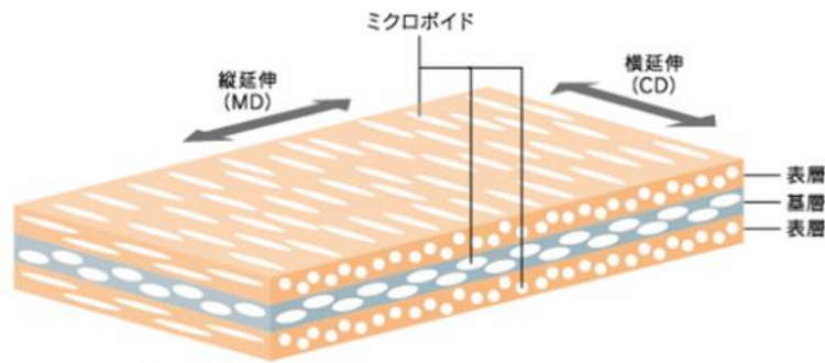
図-2：ユポの構造図
